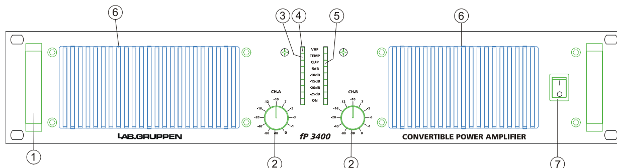
Figure 1 : Panneau avant
