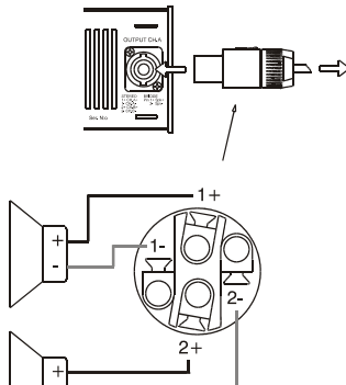
Canal A et canal B dans un seul connecteur Speakon (Stéréo et Bi-amp)
