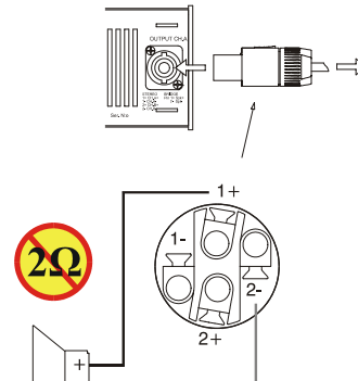
Branchement bridgé
